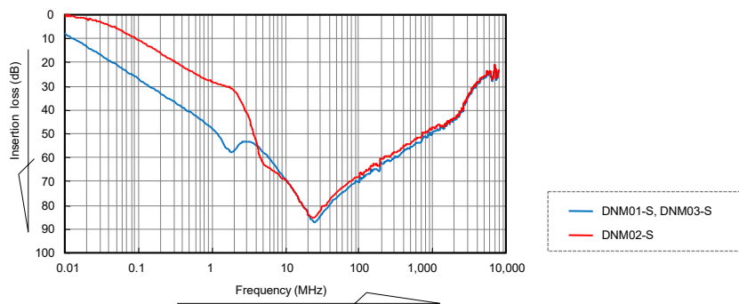
挿入損失特性(参考)
