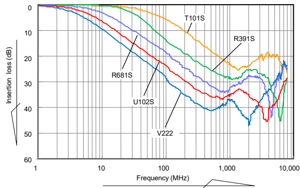
挿入損失特性(参考)
