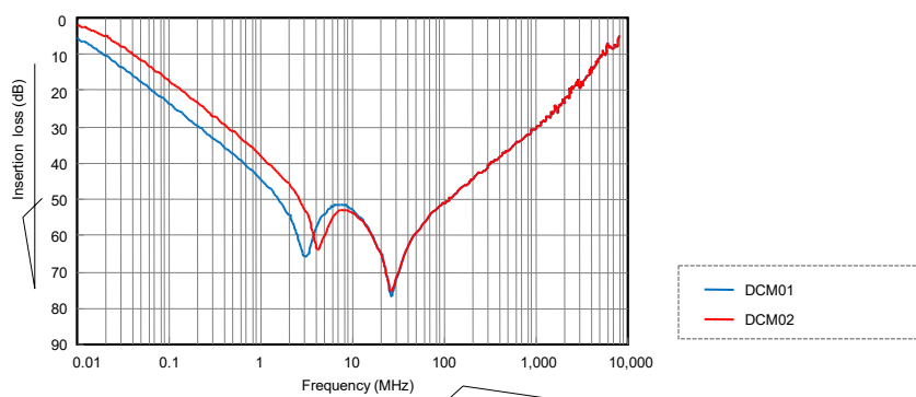
挿入損失特性(参考)
