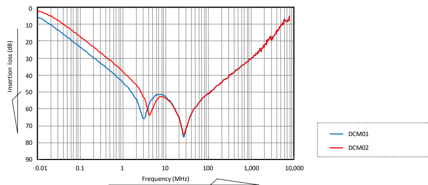
插入损耗特性 (参考)
