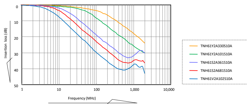
插入损失特性（参考）
